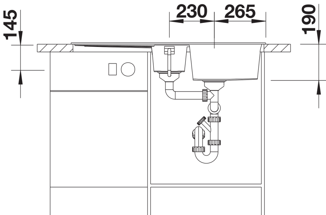
Frontansicht
