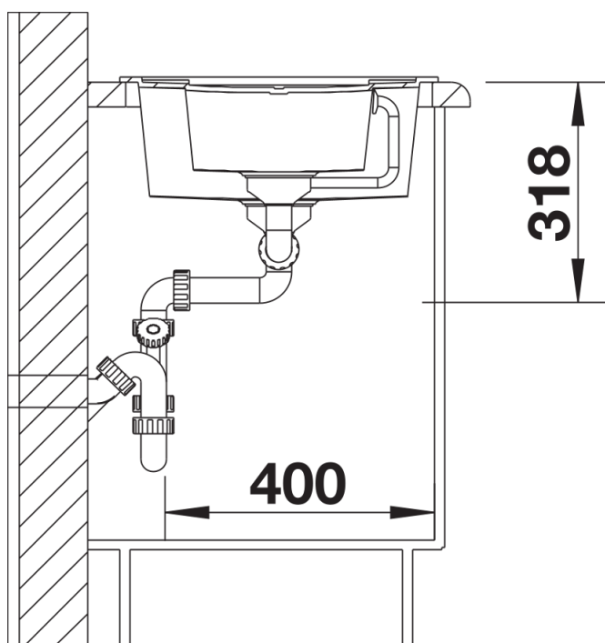
Seitenansicht
