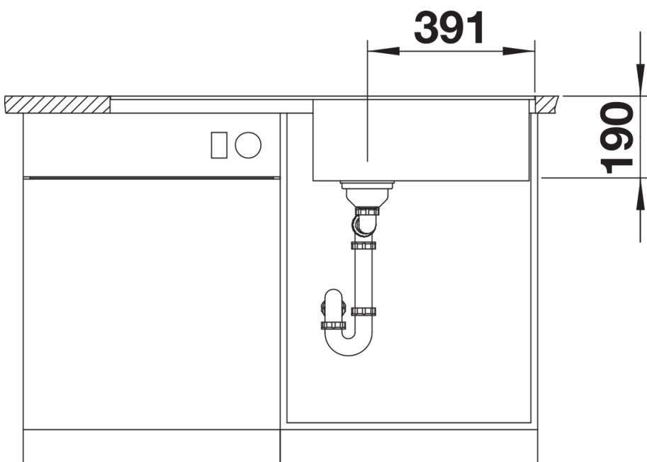
Frontansicht
