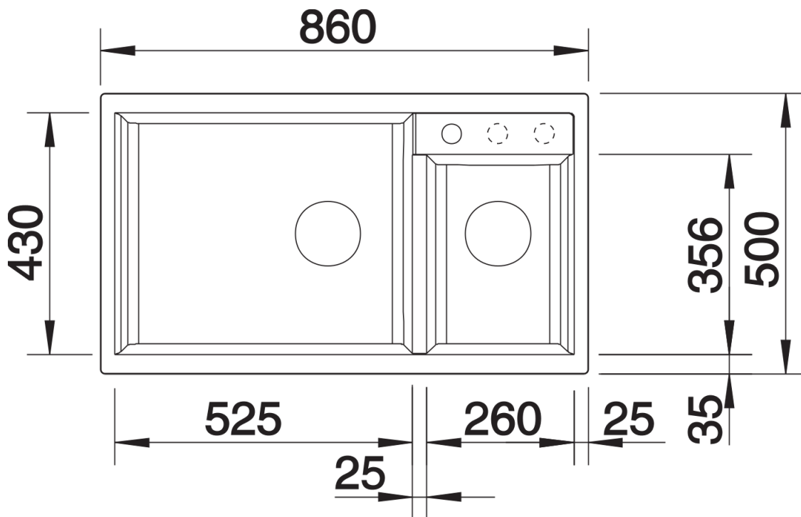
Aufsicht
