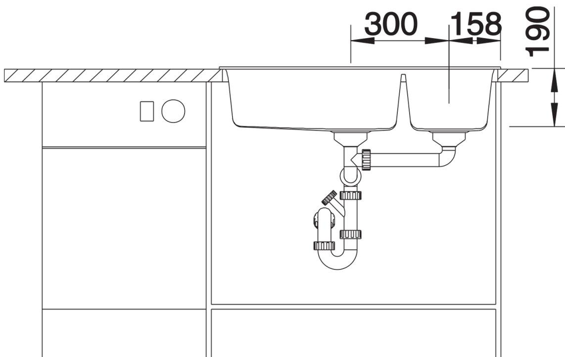
Frontansicht
