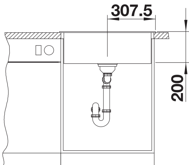
Frontansicht
