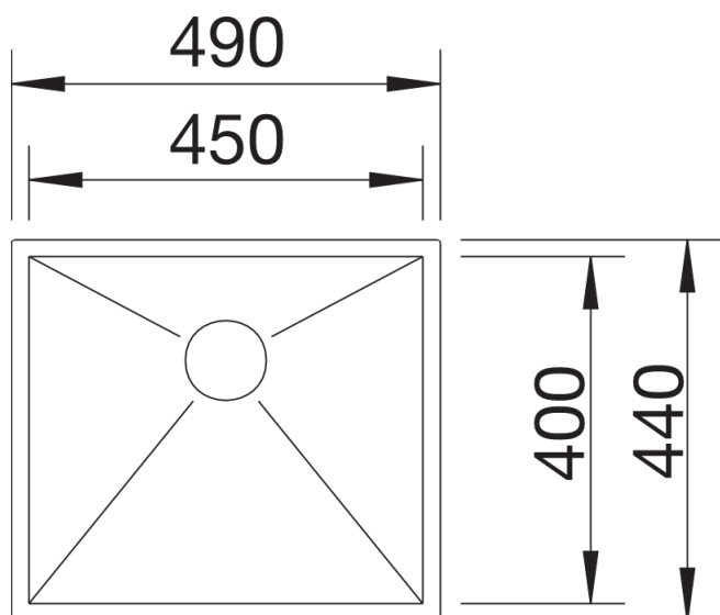
Aufsicht
