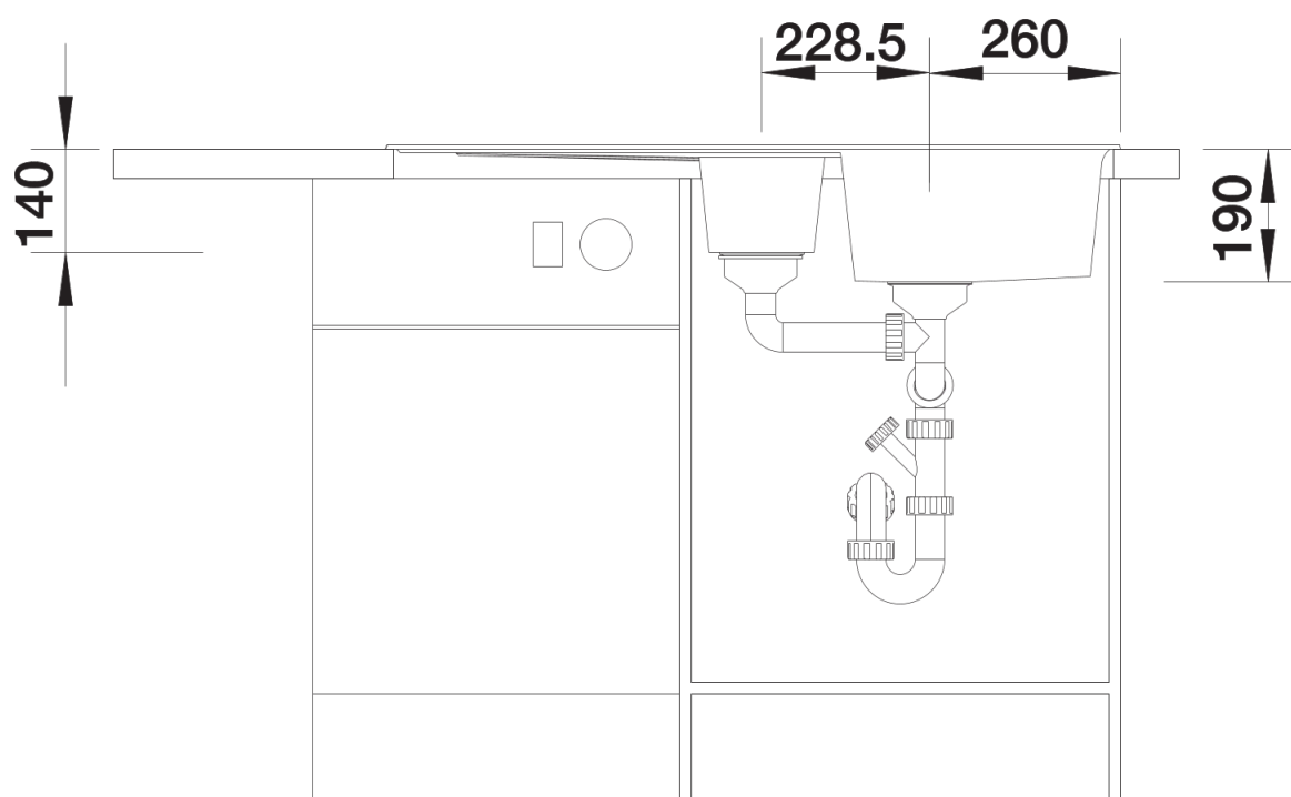
Frontansicht
