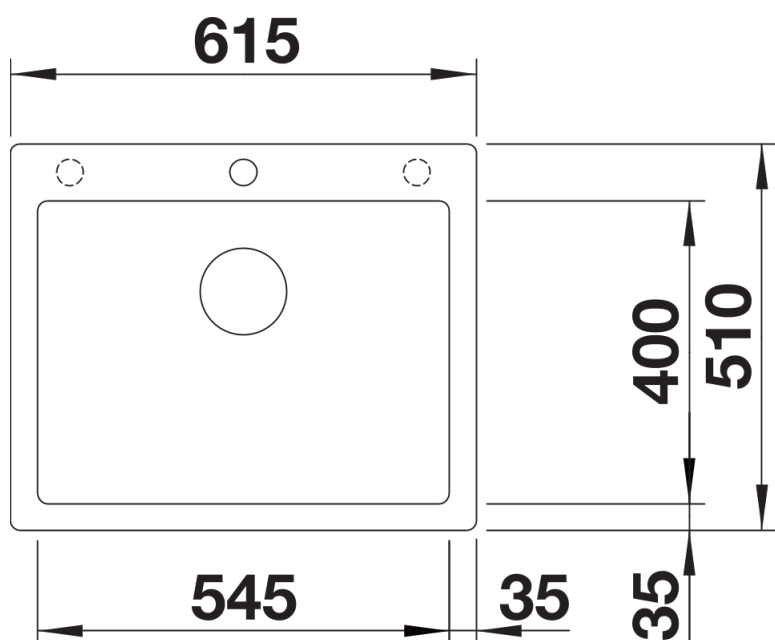
Aufsicht
