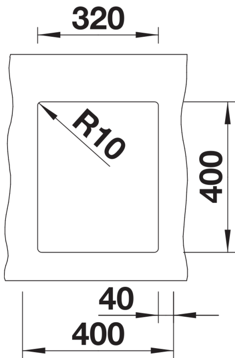
Ausschnitt
