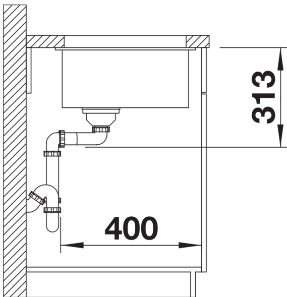
Seitenansicht
