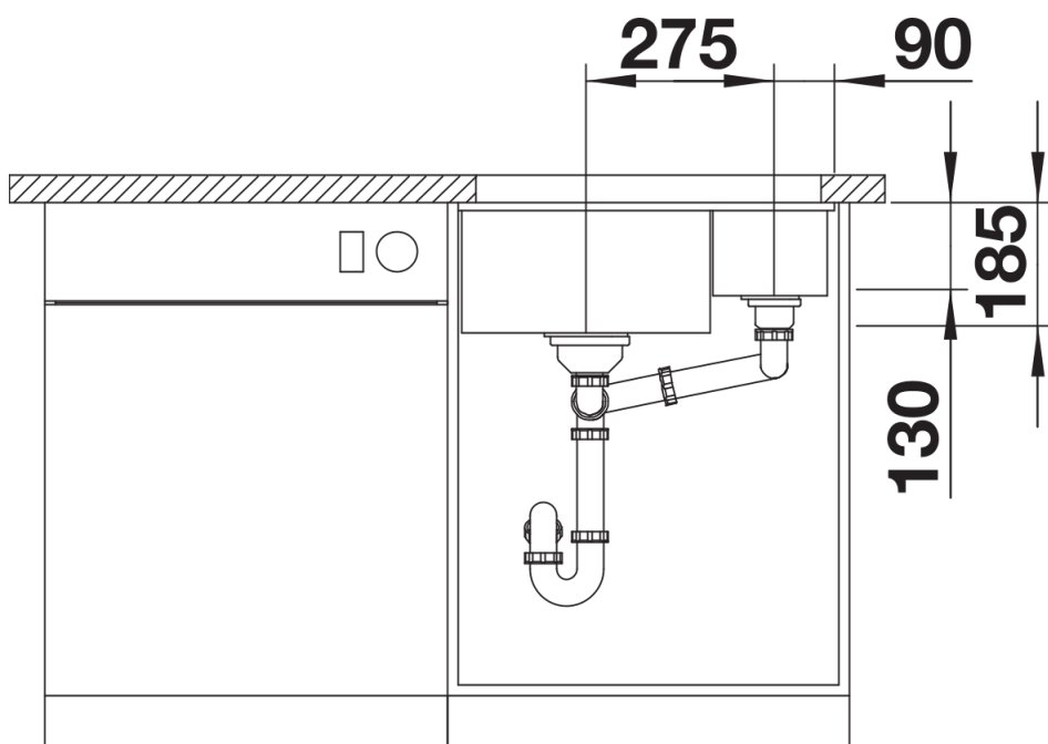
Frontansicht
