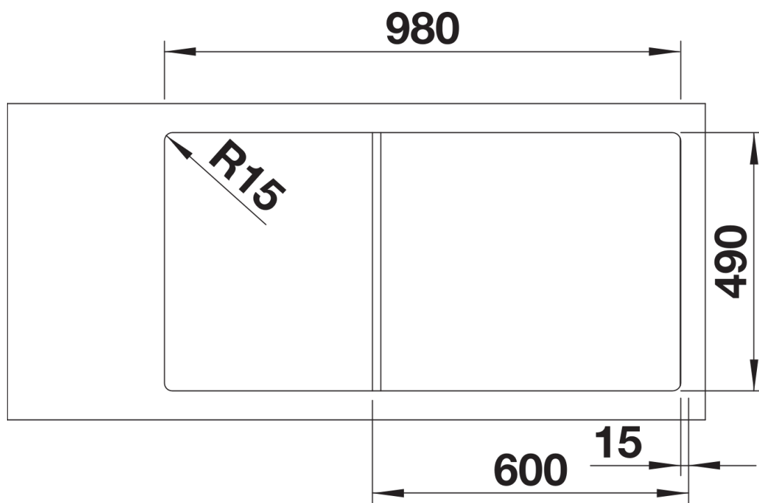
Découpe
