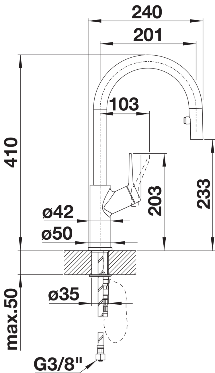
Vue latérale
