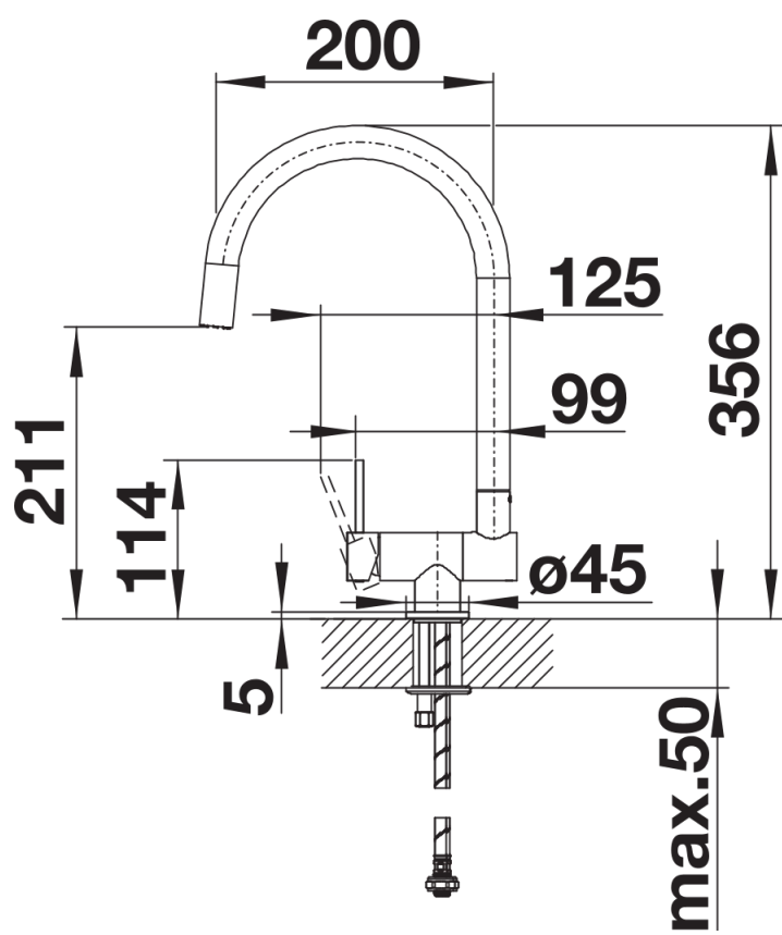
Vue latérale
