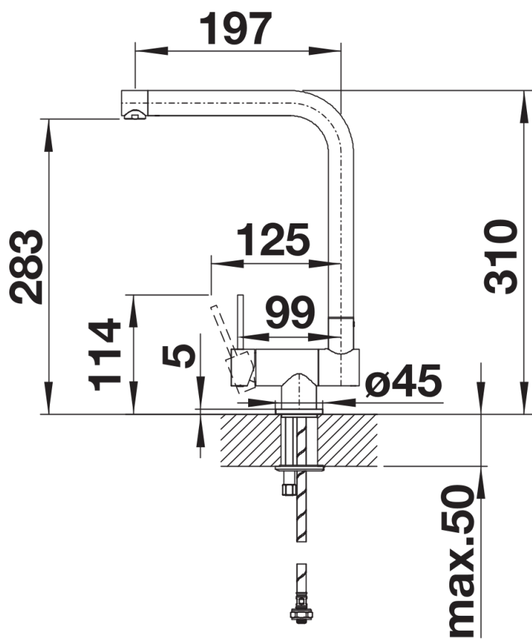
Vue latérale
