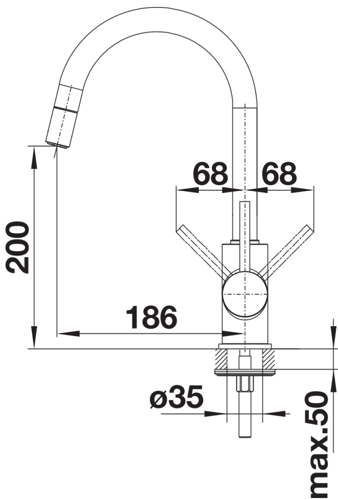
Vue latérale
