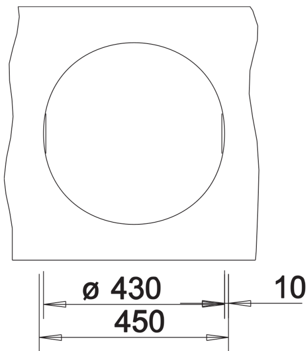
Découpe
