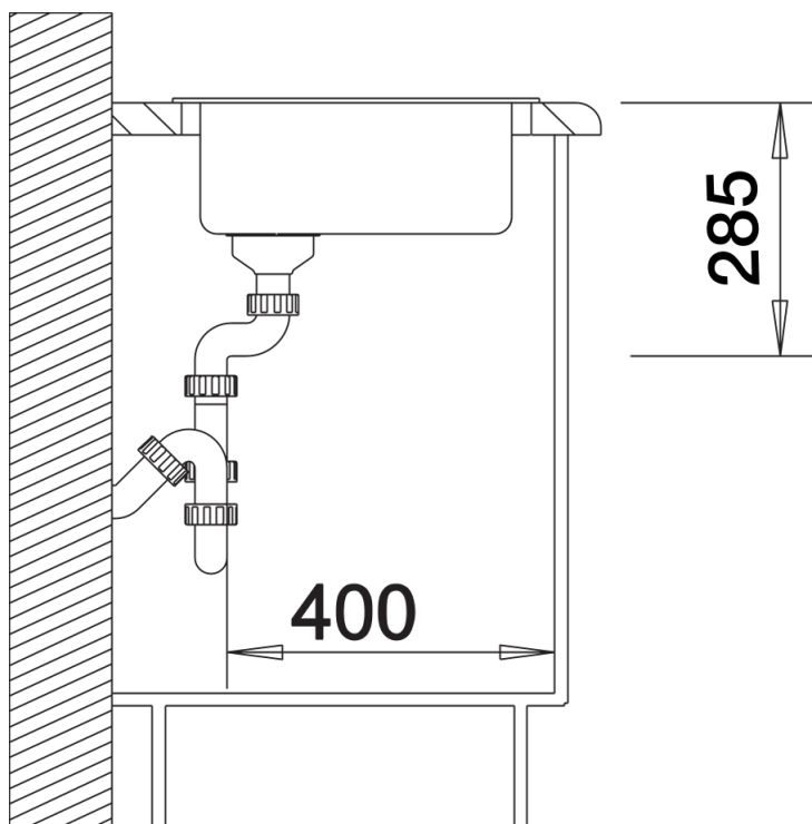
Vue latérale
