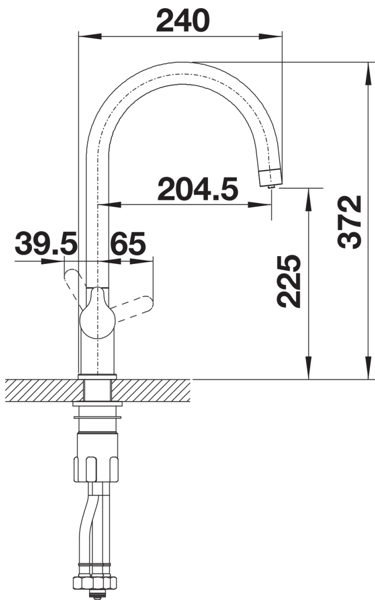
Vue latérale
