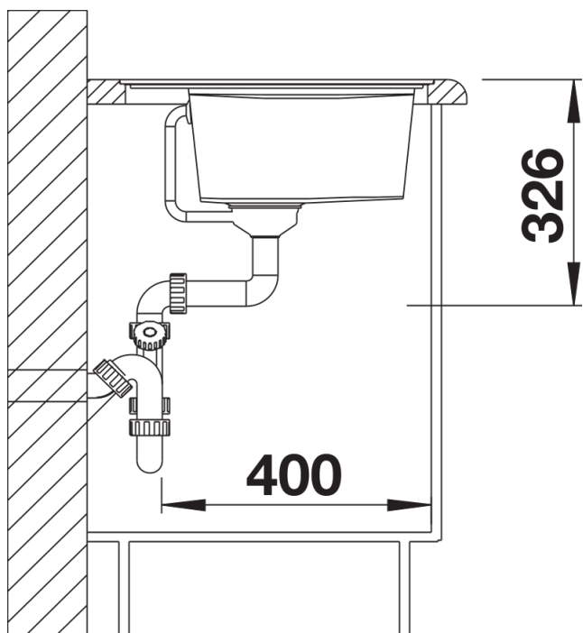
Vue latérale
