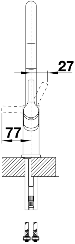
Swivel range
