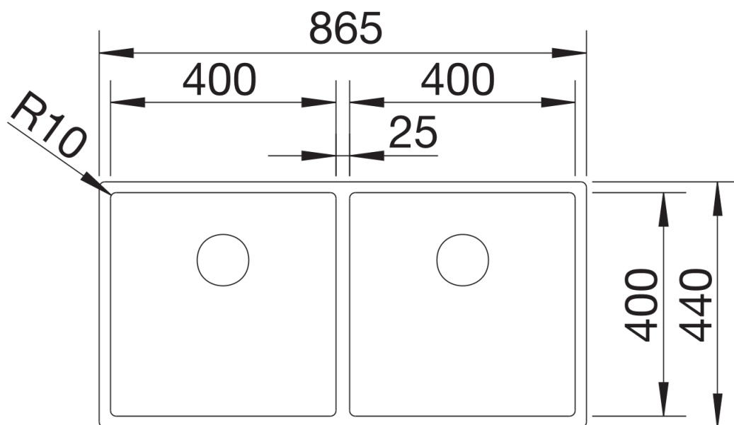
Felülnézet
