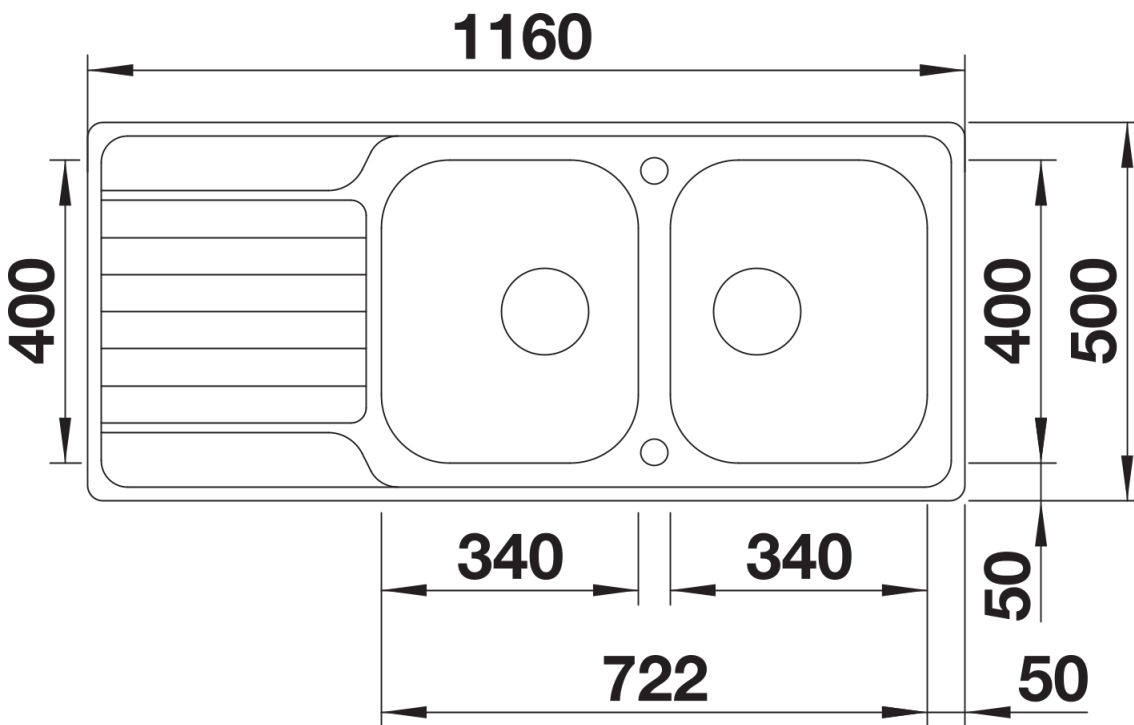
Vista superiore
