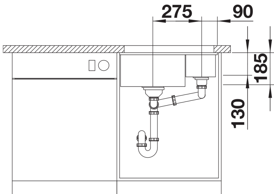
Vista frontale
