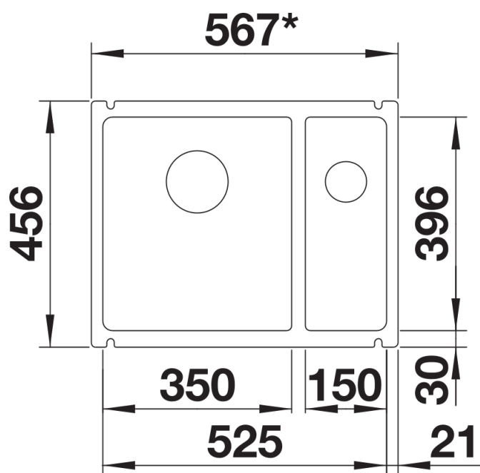
Vista superiore
