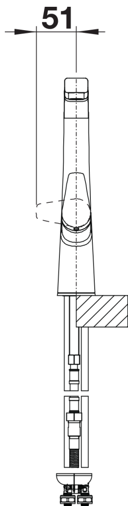
側面図ハンドギア2D
