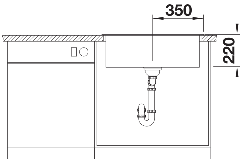
正面図
