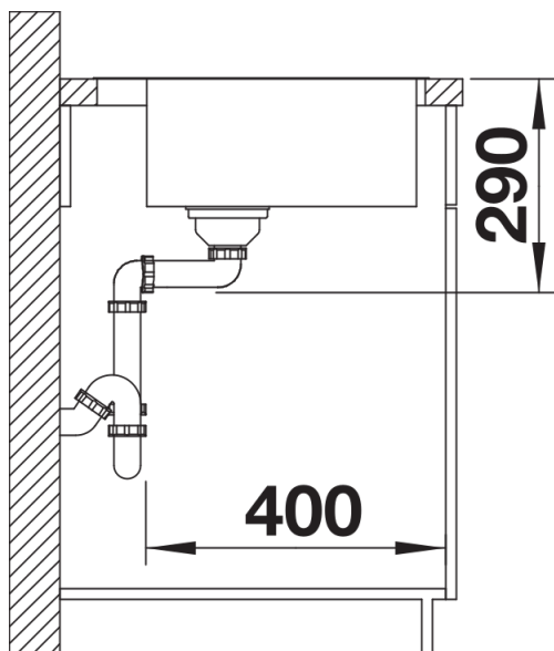
Zijaanzicht
