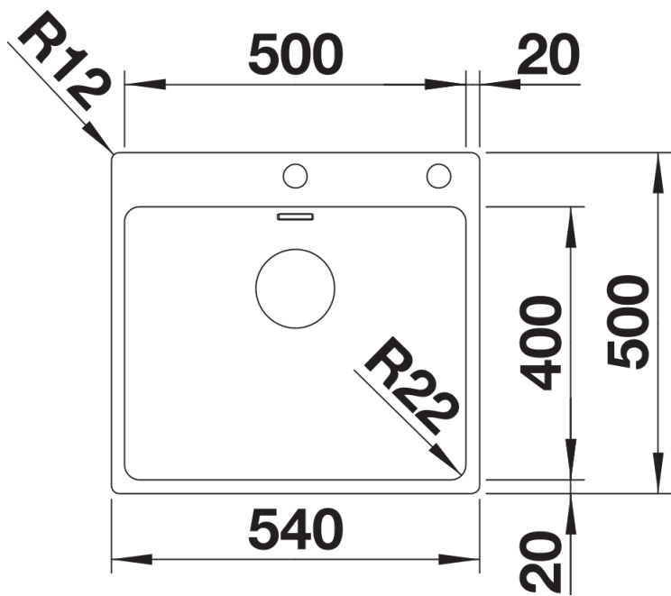
Bovenaanzicht
