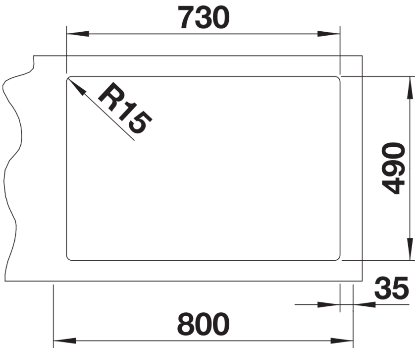
Uitgesneden
