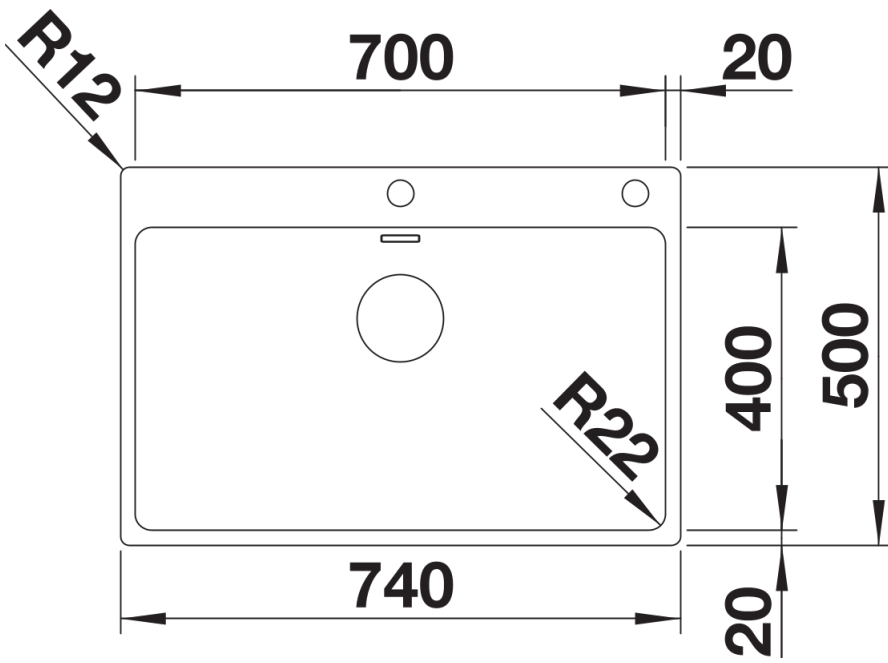
Bovenaanzicht
