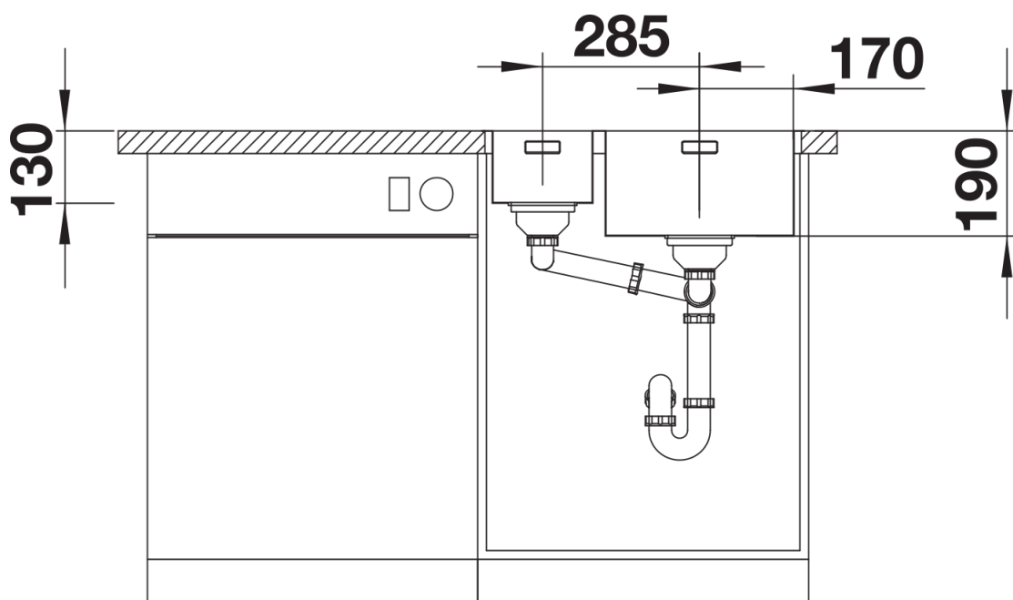
Vooraanzicht
