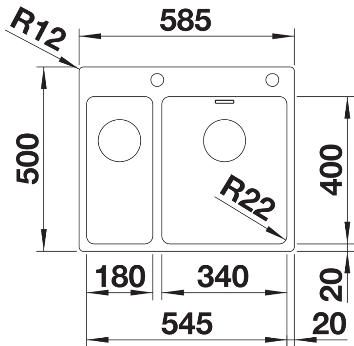
Bovenaanzicht
