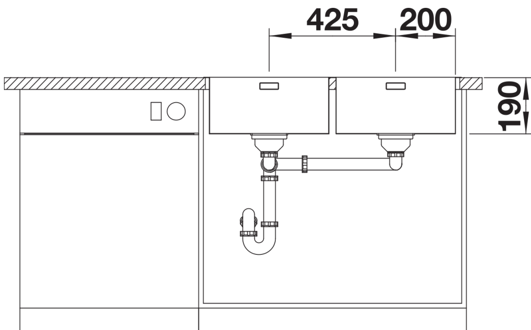
Vooraanzicht
