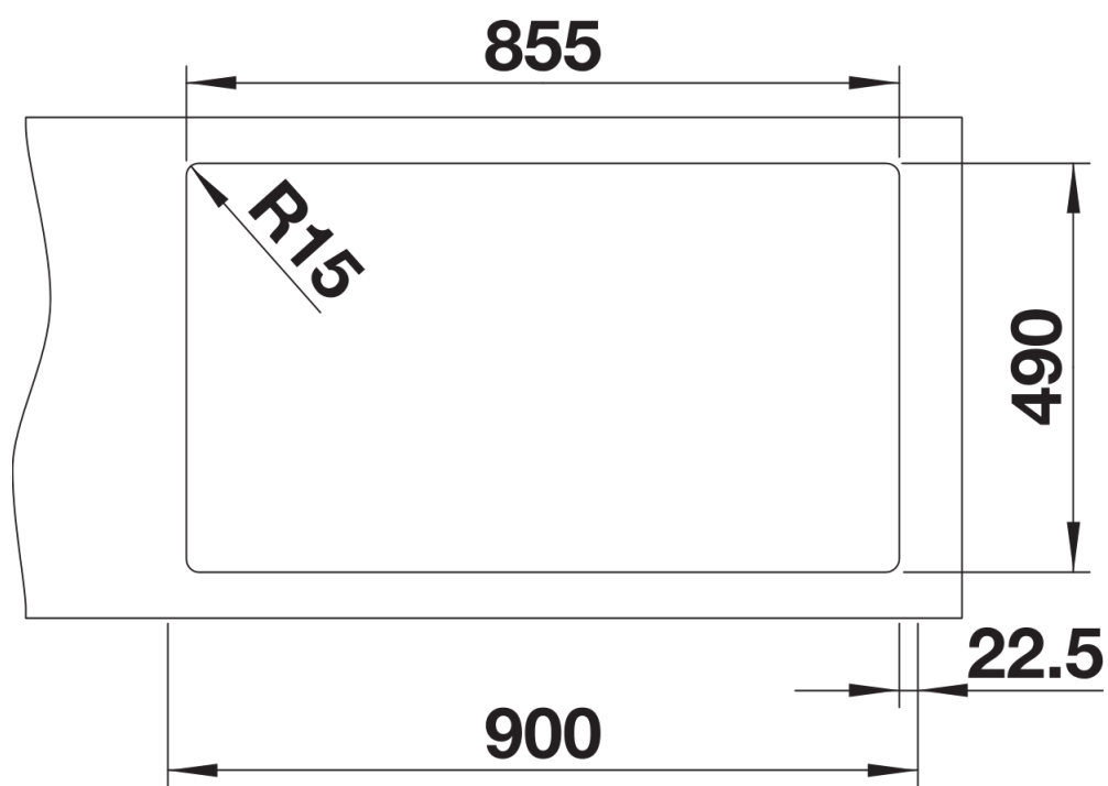
Uitgesneden
