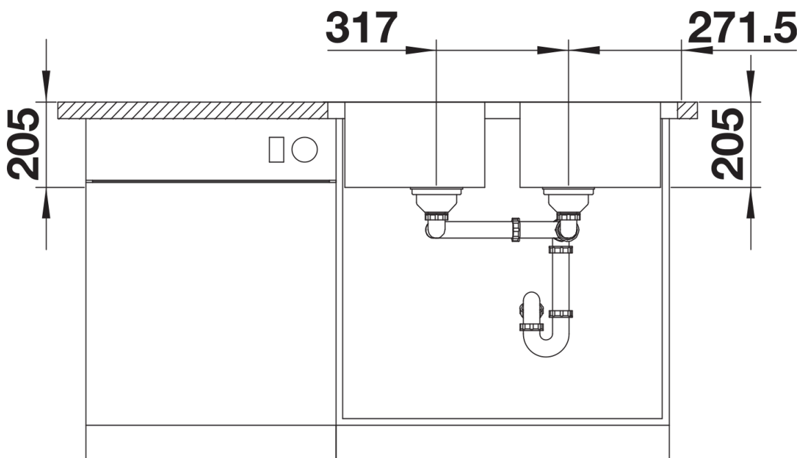
Vooraanzicht
