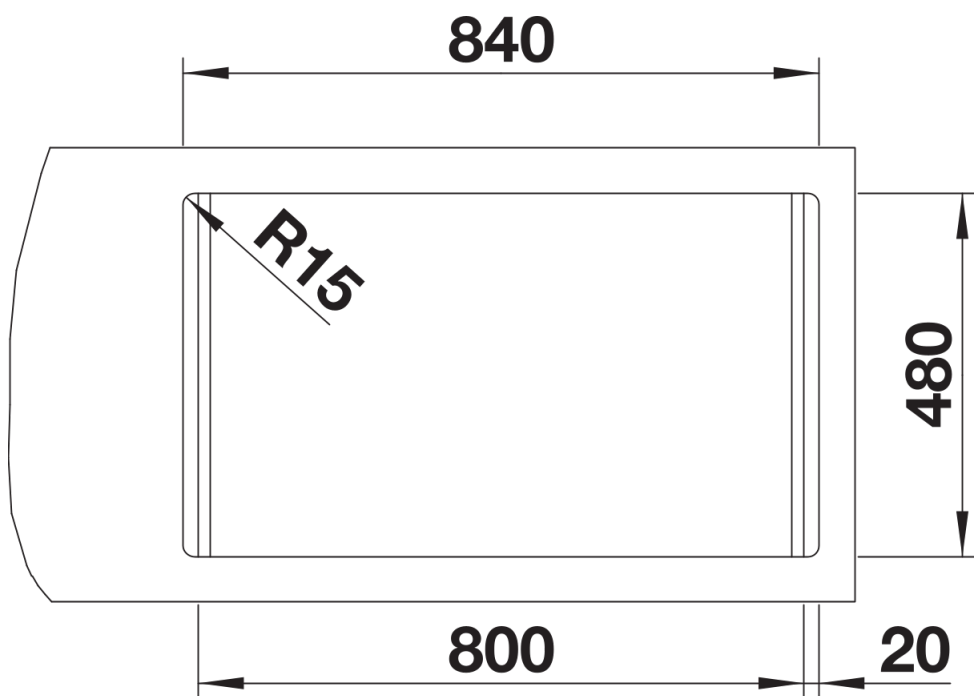
Uitgesneden
