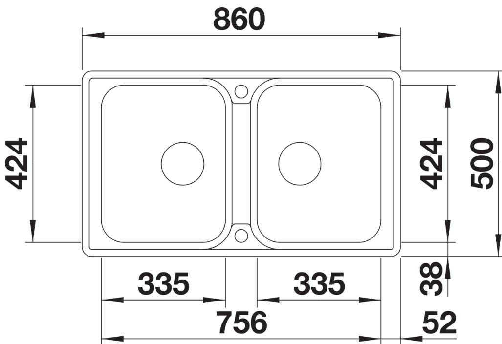
Bovenaanzicht
