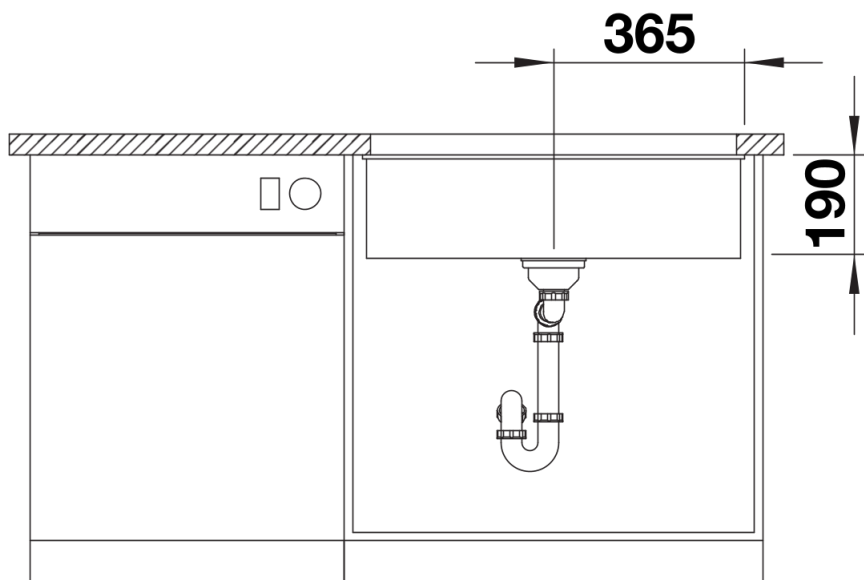
Vooranzicht
