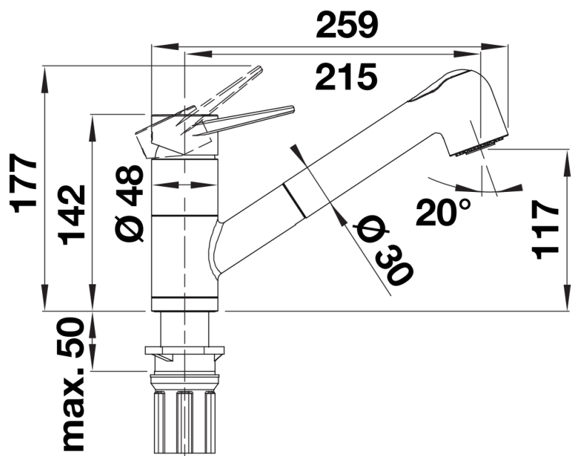
Zijaanzicht
