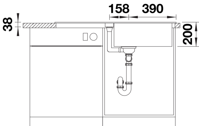
Vooraanzicht
