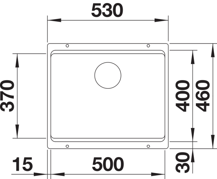
Bovenaanzicht
