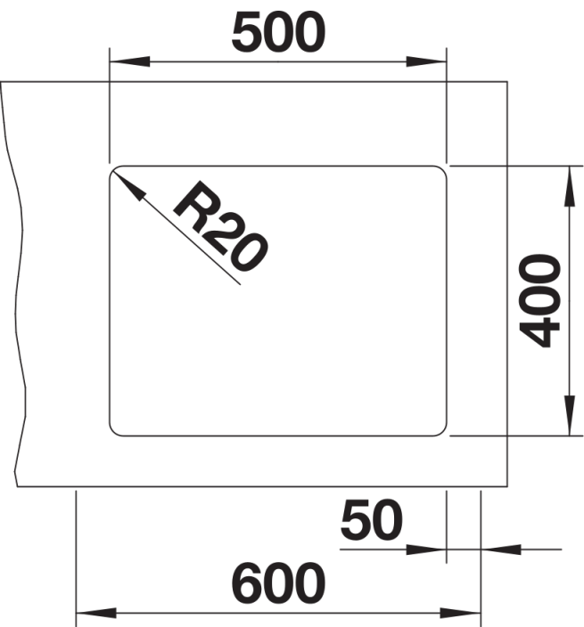
Uitgesneden
