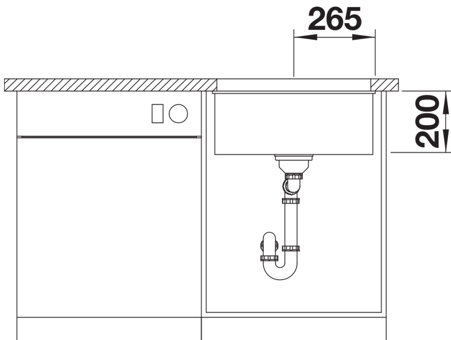
Vooraanzicht
