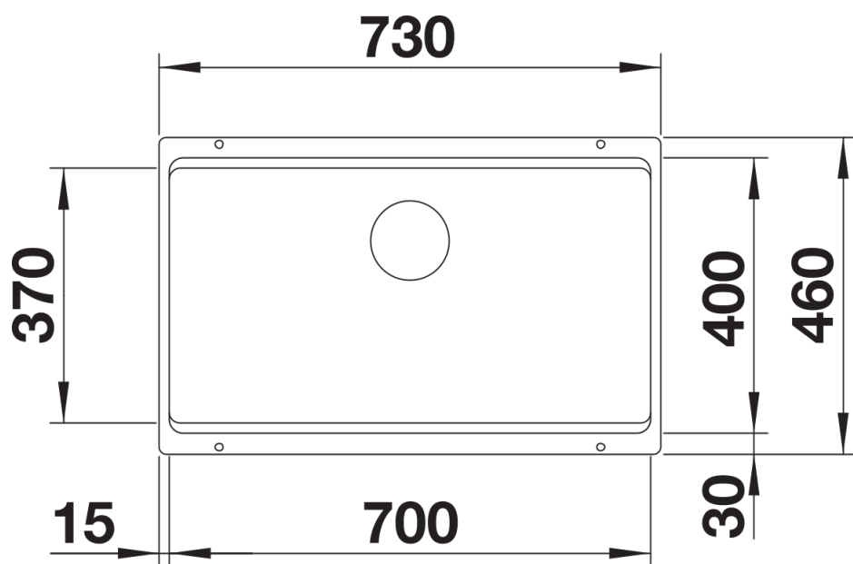
Bovenaanzicht
