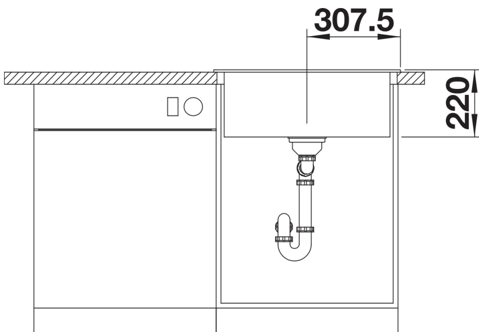
Vooraanzicht
