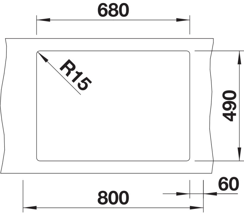
Uitgesneden
