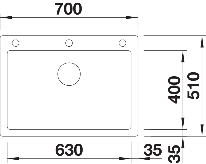
Bovenaanzicht
