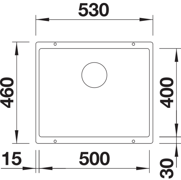
Bovenaanzicht
