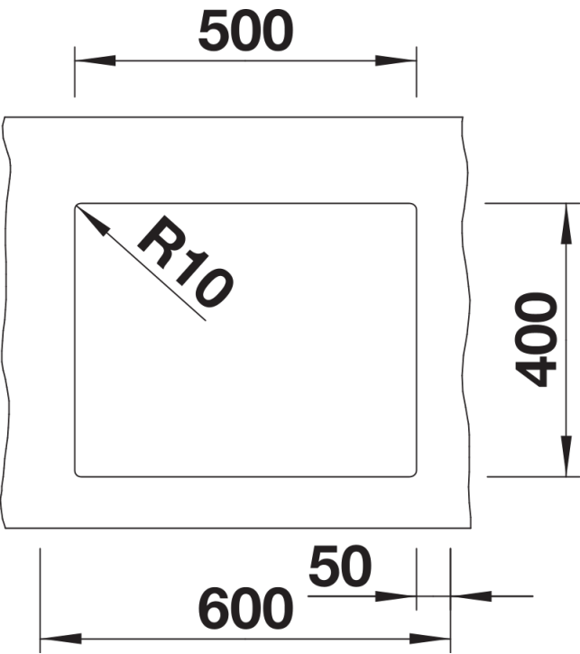
Uitgesneden
