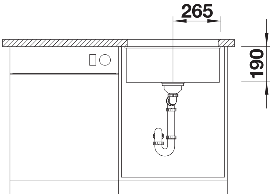
Vooraanzicht
