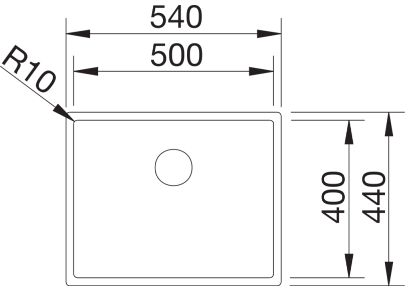
Bovenaanzicht
