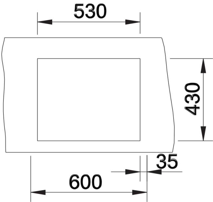
Uitgesneden
