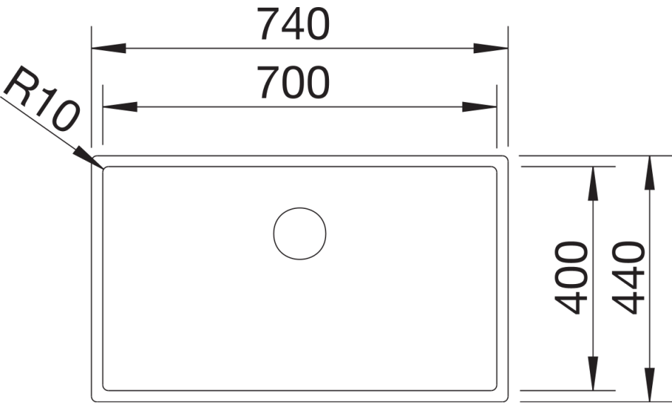
Bovenaanzicht
