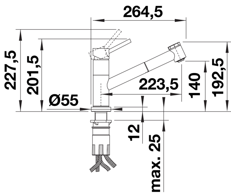
Zijaanzicht
