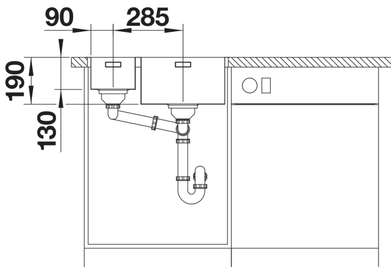
Vooraanzicht
