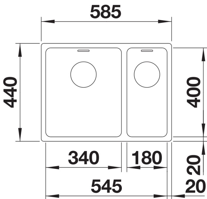
Bovenaanzicht
