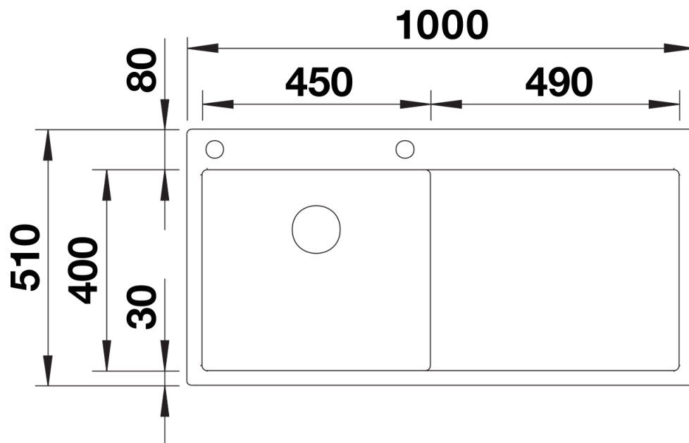
Bovenaanzicht
