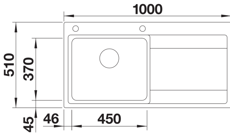
Bovenaanzicht
