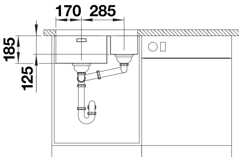
Vooraanzicht
