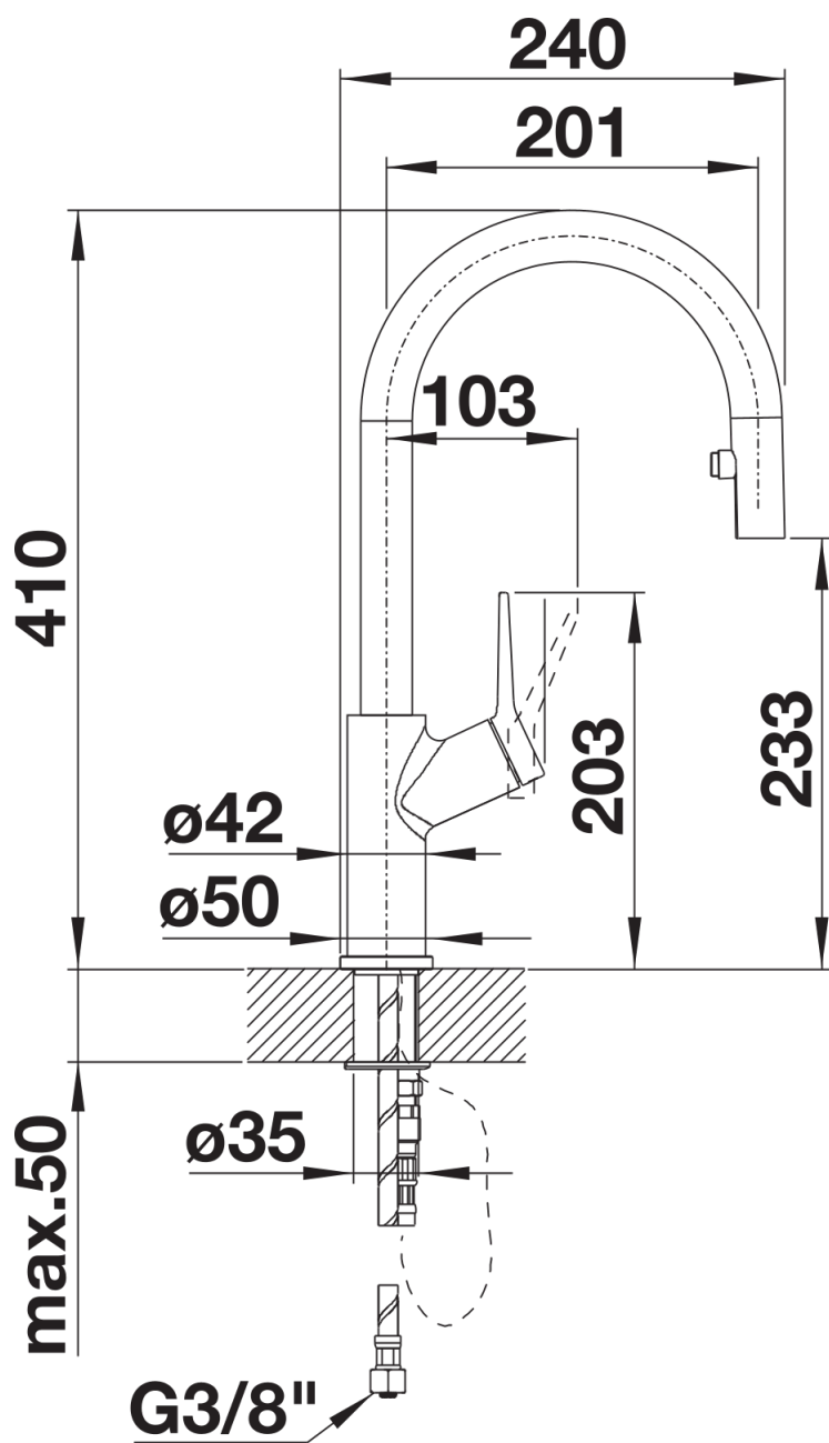
Zijaanzicht
