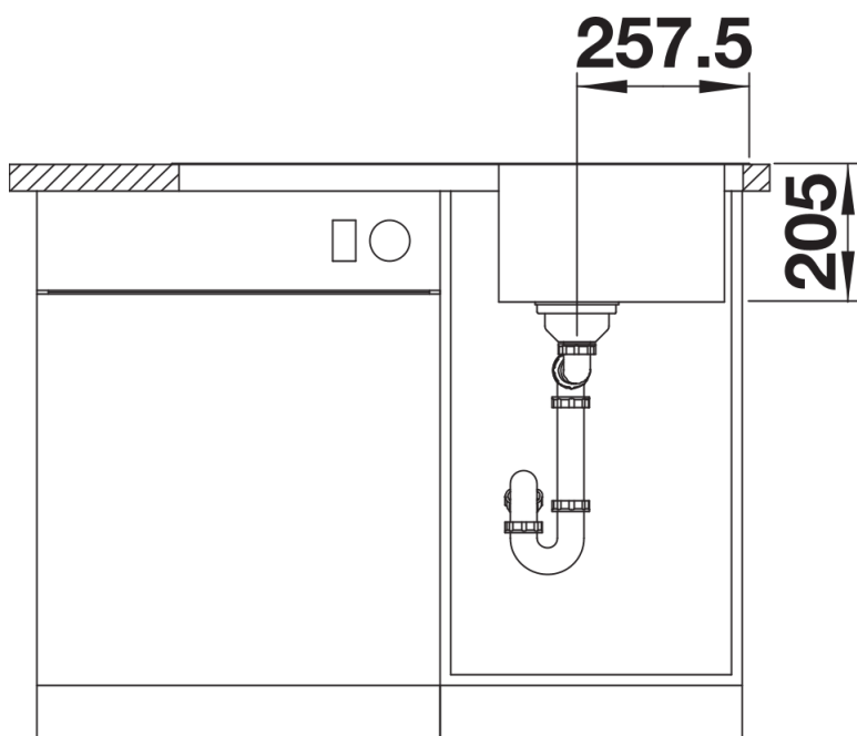
Vooraanzicht
