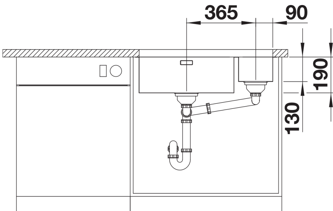
Vooraanzicht
