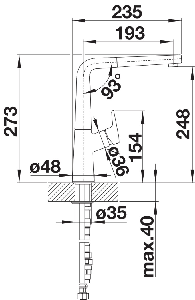
Zijaanzicht
