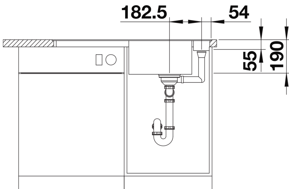
Vooraanzicht
