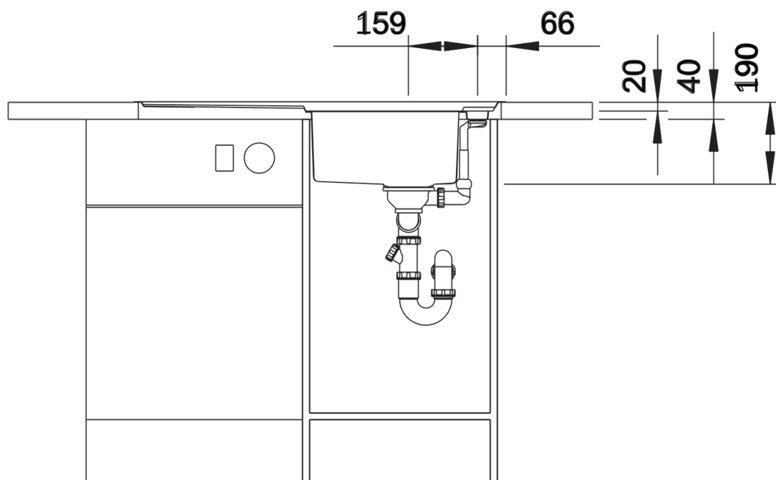
Vooraanzicht
