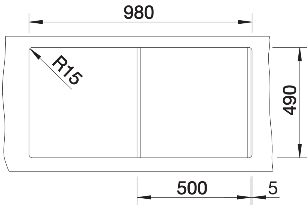
Uitgesneden
