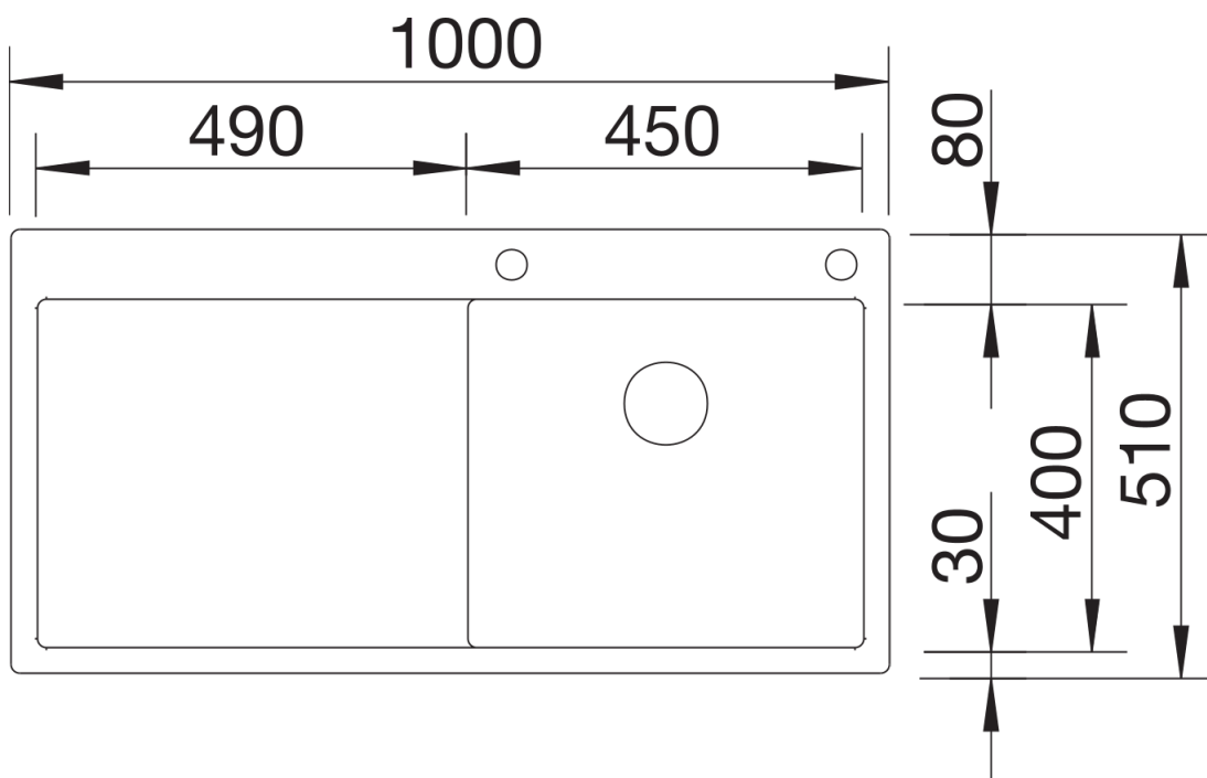
Bovenaanzicht
